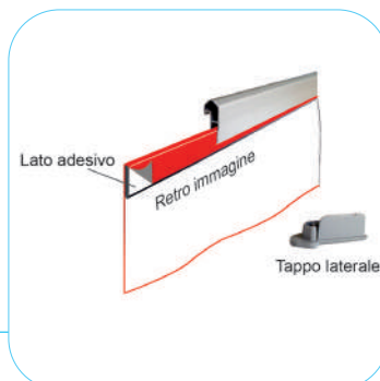
DOPPIO FISSAGGIO CON BIADESIVO
