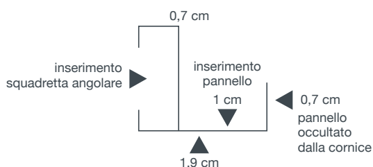
RETRO DELLA CORNICE
